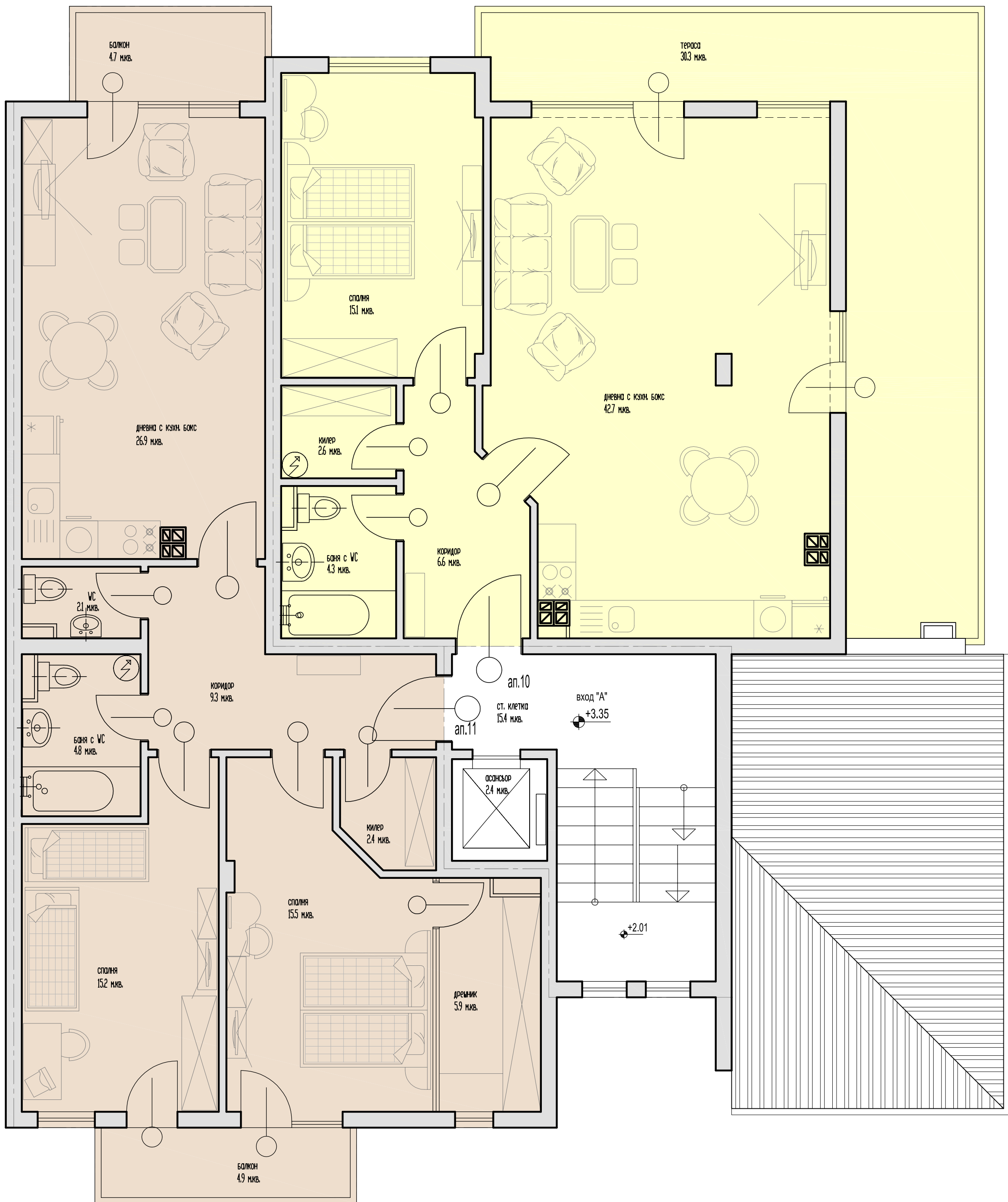
Трети етаж кота +3,35
